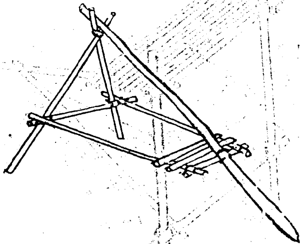
Kiểu sàn không cần dây néo
